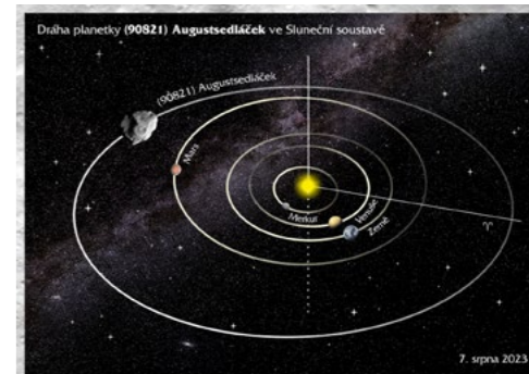
Dráha planetky Augustsedláček
